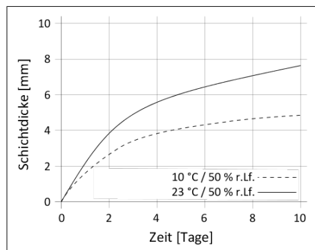
Diagramm 1: Durchhärtegeschwindigkeit Sikaflex®-529 Evolution
